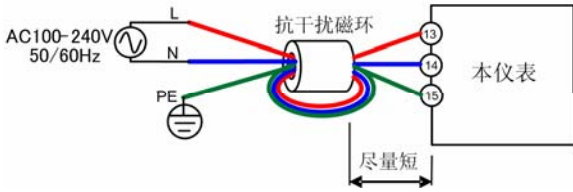
抗干扰磁环安装示意图
